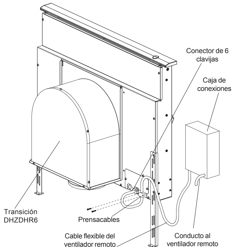
Figura 11 - Ventilador remoto
