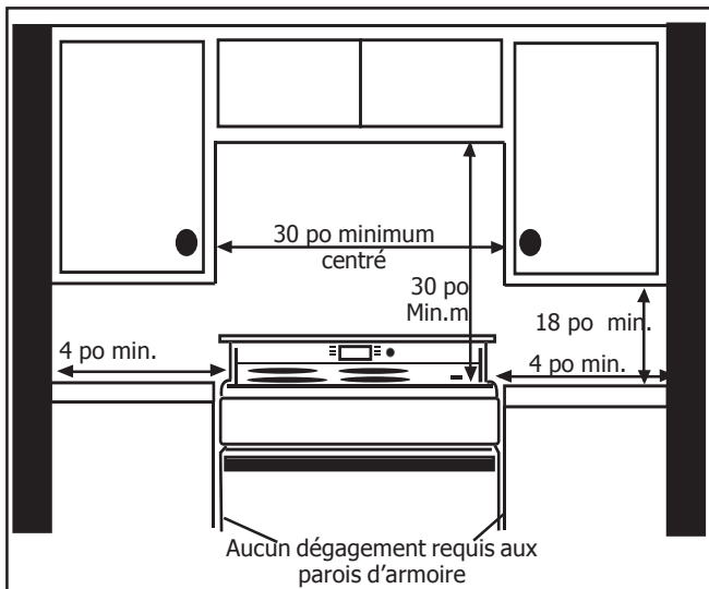
Figure 1: Préparation d'armoire
