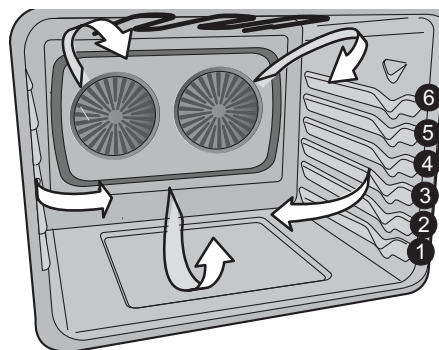
Figure 15 : Circulation d'air de rôtissage à convection et positions des grilles
