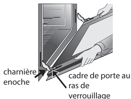
Figure 37 : Position de retrait de la porte
