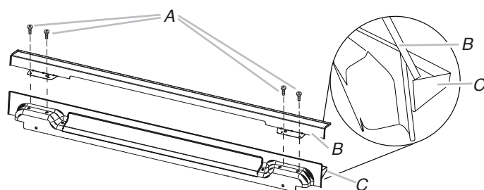
A. Vis n° 8-18 x 1/4" B. Déflecteur pour tiroir-réchaud C. Évent
