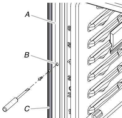
A. Châssis du four B. Trou du châssis du four C. Garniture noire
