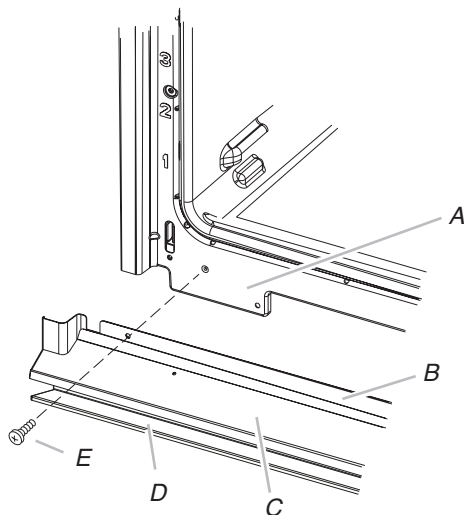
A. Châssis du four B. Onglet de l'évent C. Évent du four D. Déflecteur pour tiroir-réchaud E. Vis n° 8-18 x 3/8"
