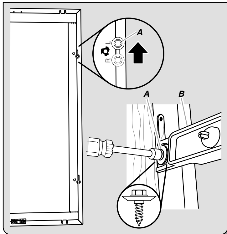
A. Arandela de tope y tornillo puntiagudo de cabeza hexagonal B. Bloque de instalación
