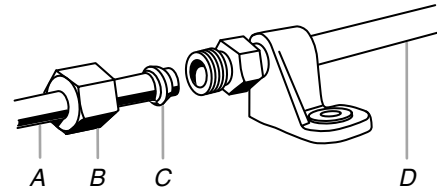
A. Tubería a la fábrica de hielo C. Férrula (comprada) B. Tuerca (comprada) D. Línea provista de la fábrica de hielo
