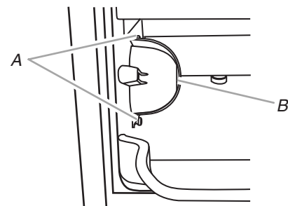
A. Tornillo de mariposa B. Soporte de la pala para el hielo
