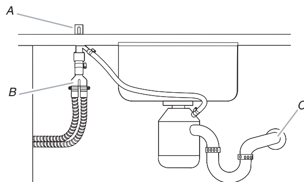
A. Raccord du tuyau de vidange B. Dispositif anti-refoulement C. Déchets
