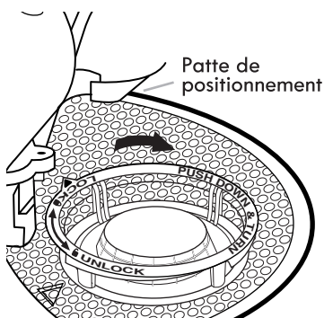
Réinstallation du filtre supérieur
