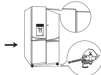
5 Nivelación y alineación de las puertas
