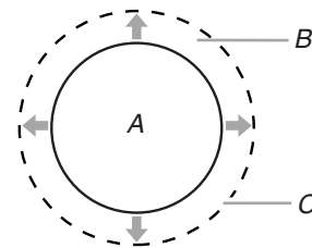
A. Zone de cuisson à la surface B. Ustensiles de cuisson/autoclave C. Dépassement maximum de \frac{1}{2} " (1,3 cm)
