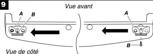
A. Butée de la porte B. Vis de butée de la porte
