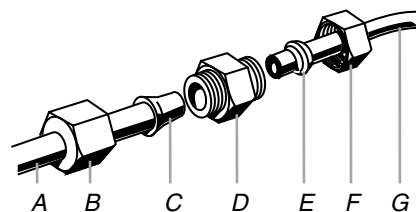
A. Tube vers le réfrigérateur B. Écrou (fourni) C. Renflement D. Raccord (fourni) E. Virole (à acheter) F. Écrou (à acheter) G. Canalisation d'eau du domicile
