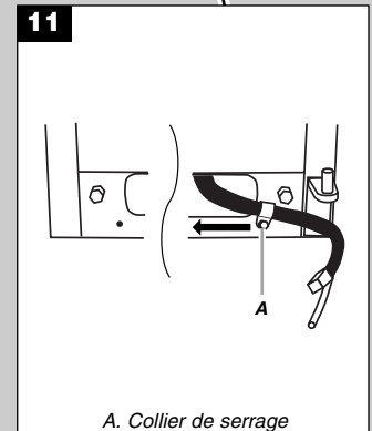
A. Collier de serrage
