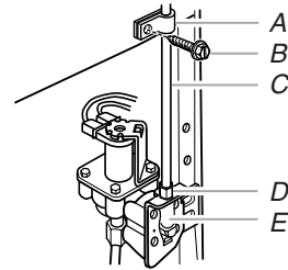
A. Abrazadera para tubería B. Tornillo de abrazadera C. Tubería de cobre D. Tuerca de compresión para tubería E. Entrada de la válvula
