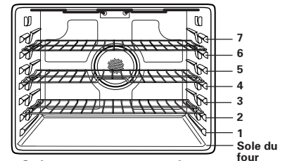
Cuisson avec convection sur trois grilles
