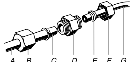
A. Conduit vers le réfrigérateur B. Écrou (fourni) C. Renflement D. Raccord (à acheter) E. Virole (à acheter) F. Écrou (à acheter) G. Canalisation d'eau du domicile
