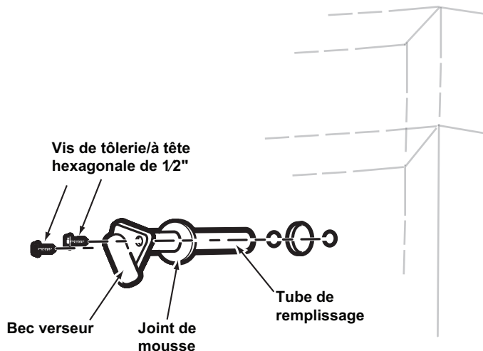
Installation de l'ensemble tube de remplissage/joint (Modèles à congélateur en bas - 14 à 18 pi³)
