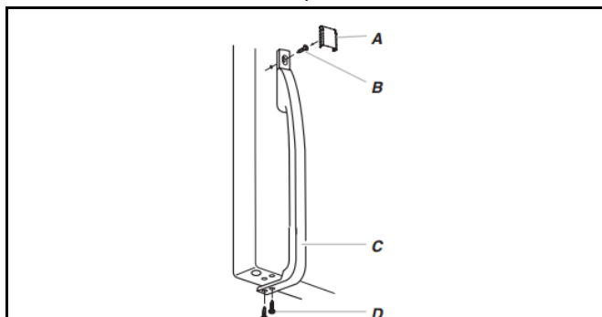
A. Cache-vis C. Poignée du congélateur B. Vis de poignée D. Vis de poignée à tête plate
