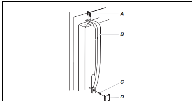
A. Vis de poignée à tête plate C. Vis de poignée B. Poignée du réfrigérateur D. Cache-vis
