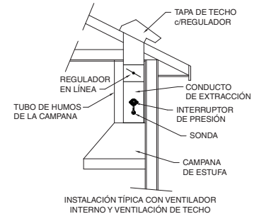
INSTALACIÓN TÍPICA CON VENTILADOR INTERNO Y VENTILACIÓN DE TECHO
