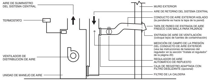
Regulador conectado al lado de retorno del sistema de conducto central.
