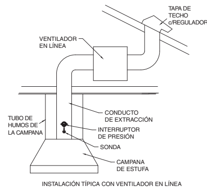
INSTALACIÓN TÍPICA CON VENTILADOR EN LÍNEA
