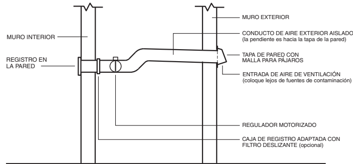
Regulador conectado con conductos de aire exterior directamente a un cielo raso, piso o registro de pared.
