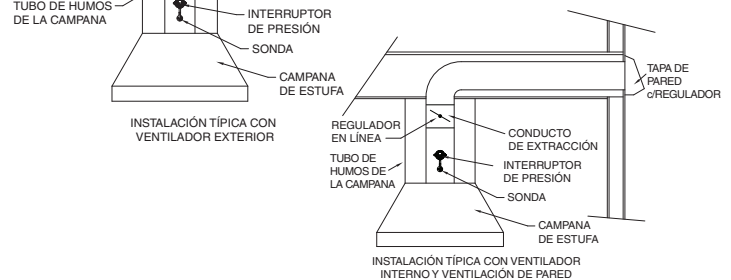
INSTALACIÓN TÍPICA CON VENTILADOR INTERNO Y CONDUCTOS HORIZONTALES CON VENTILACIÓN DE PARED
