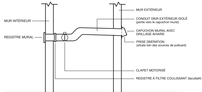
Clapet et conduit extérieur raccordés directement au registre d'un plafond, d'un mur ou d'un plancher.
