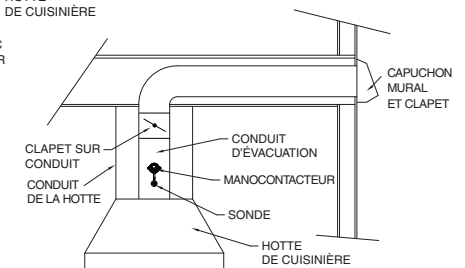
INSTALLATION TYPE AVEC VENTILATEUR INTERNE ET ÉVENT MURAL
