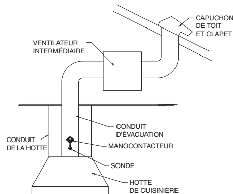
INSTALLATION TYPE AVEC VENTILATEUR INTERMÉDIAIRE
