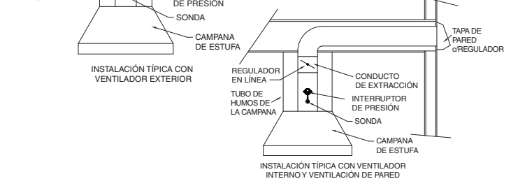
INSTALACIÓN TÍPICA CON VENTILADOR INTERNO Y CONDUCTOS HORIZONTALES CON VENTILACIÓN DE PARED
