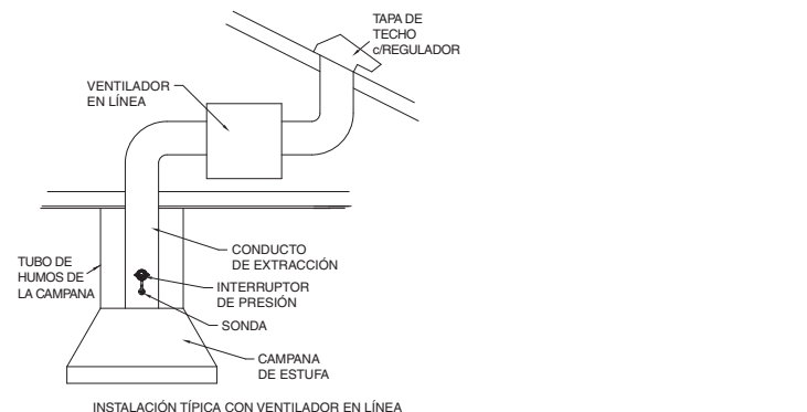
INSTALACIÓN TÍPICA CON VENTILADOR EN LÍNEA
