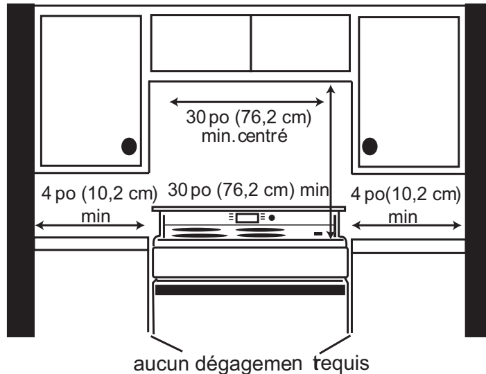
Figure 7: Préparation de l'armoire
