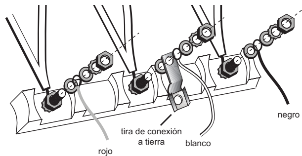
Figura 17: Conexión de 3 hilos
