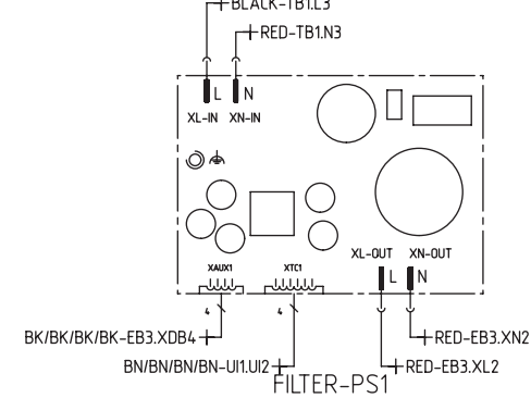
Unidad de alimentación
