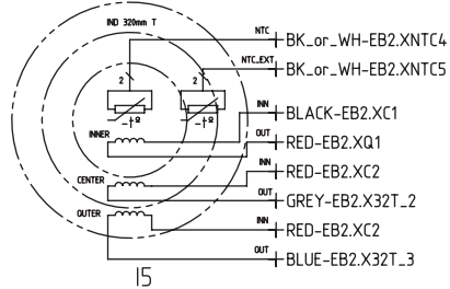
Bobina de inducción
