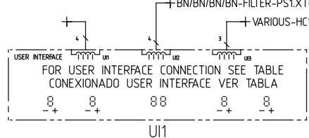
Placa electrónica de mando
