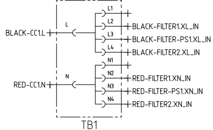
Bloque de terminales
