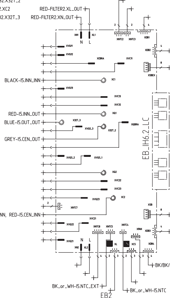
Unidad electrónica de potencia
