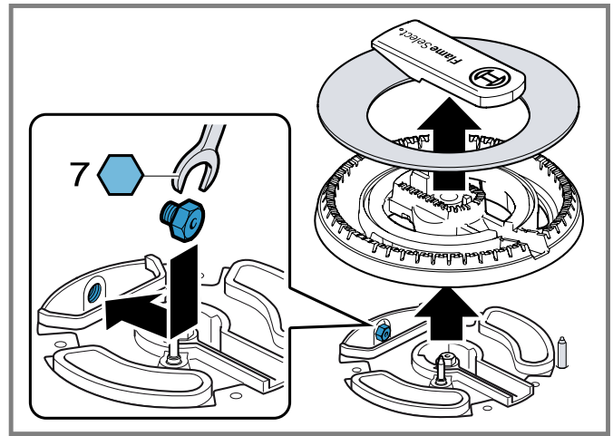
Quemador de doble llama, primera esprea
