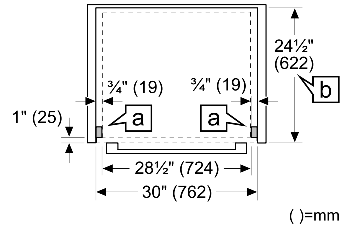
Puerta con bisagra inferior, vista superior
