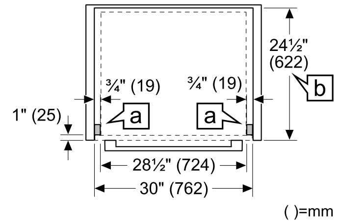
Vue de dessus porte à charnières inférieure
