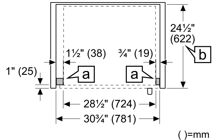
Vue de dessus porte battante gauche
