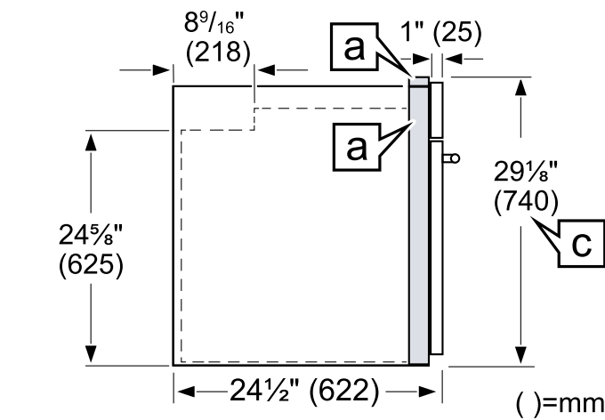
Vista lateral (representativa)
