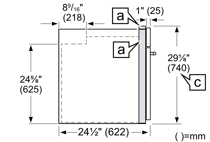
Vue latérale (représentative)
