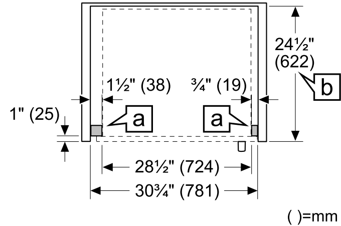
Puerta con bisagra a la izquierda, vista superior
