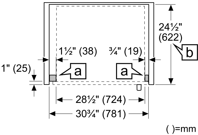
Top view left swing door
