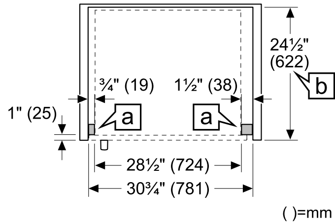
Puerta con bisagra a la derecha, vista superior
