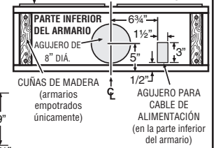
CONDUCTO REDONDO DE 7" PARTE DELANTERA DEL ARMARIO
