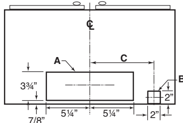
CAMPANA CON UN SOLO VENTILADOR INTERIOR
