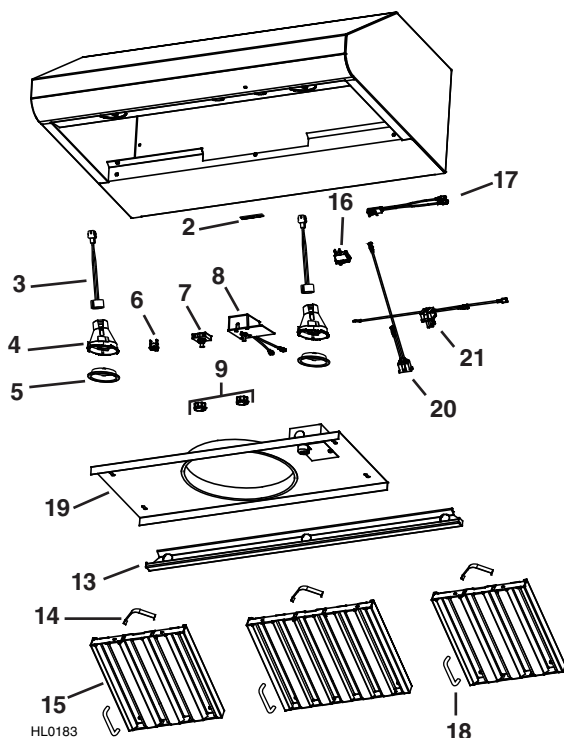
Broan Elite Série E64000 Hotte à ventilateur extérieur ou en ligne
