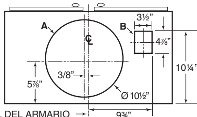
CAMPANA CON VENTILADOR EN LÍNEA O EXTERIOR VISTA INFERIOR DEL ARMARIO
