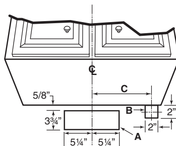
CAMPANA CON VENTILADOR EN LÍNEA O EXTERIOR VISTA INFERIOR DEL ARMARIO
