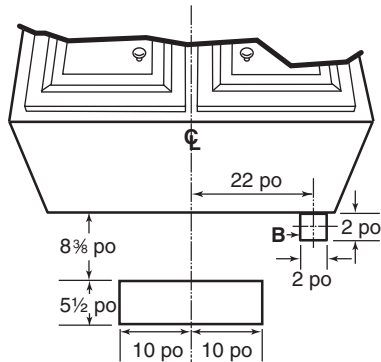
HOTTE À VENTILATEUR INTERNE DOUBLE
