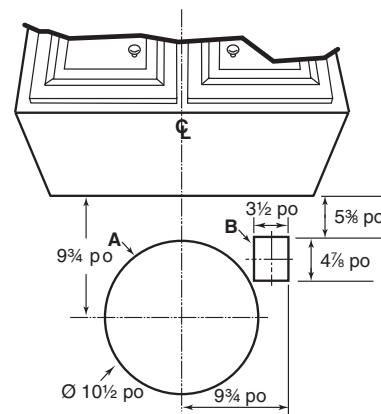
HOTTE AVEC VENTILATEUR EN LIGNE OU EXTÉRIEUR
