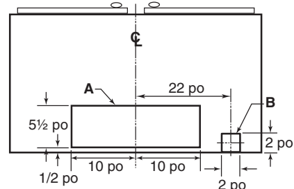
HOTTE À VENTILATEUR INTERNE DOUBLE
