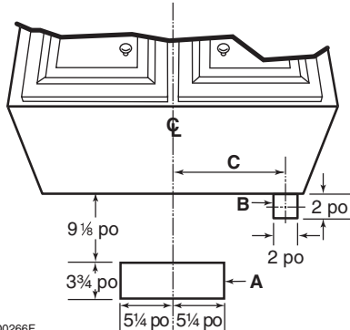
HOTTE À VENTILATEUR INTERNE SIMPLE
