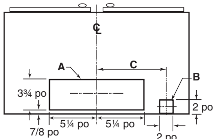
HOTTE À VENTILATEUR INTERNE SIMPLE
