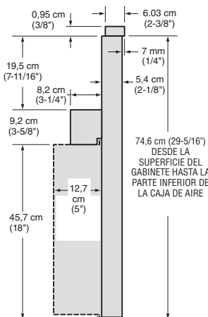
VISTA LATERAL DEL TIRO DESCENDENTE
