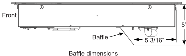
Baffle dimensions
