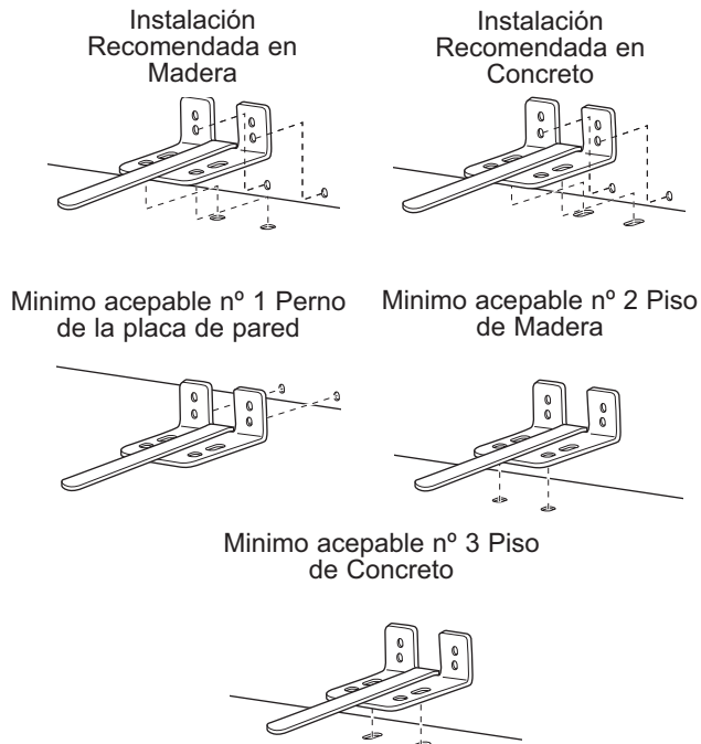
Figura 2 – Ubicaciones de tornillos aceptables
