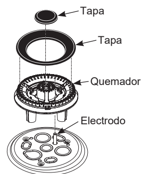
Quemador de Anillos Múltiples
