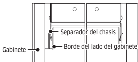
Profundidad del gabinete: 25"
