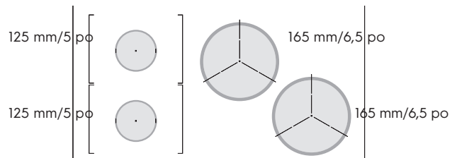
Figure 9 : Tailles de zone de cuisson, 4 zones
