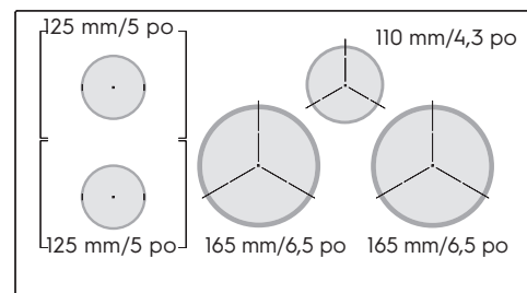
Figure 10 : Tailles de zone de cuisson, 5 zones
