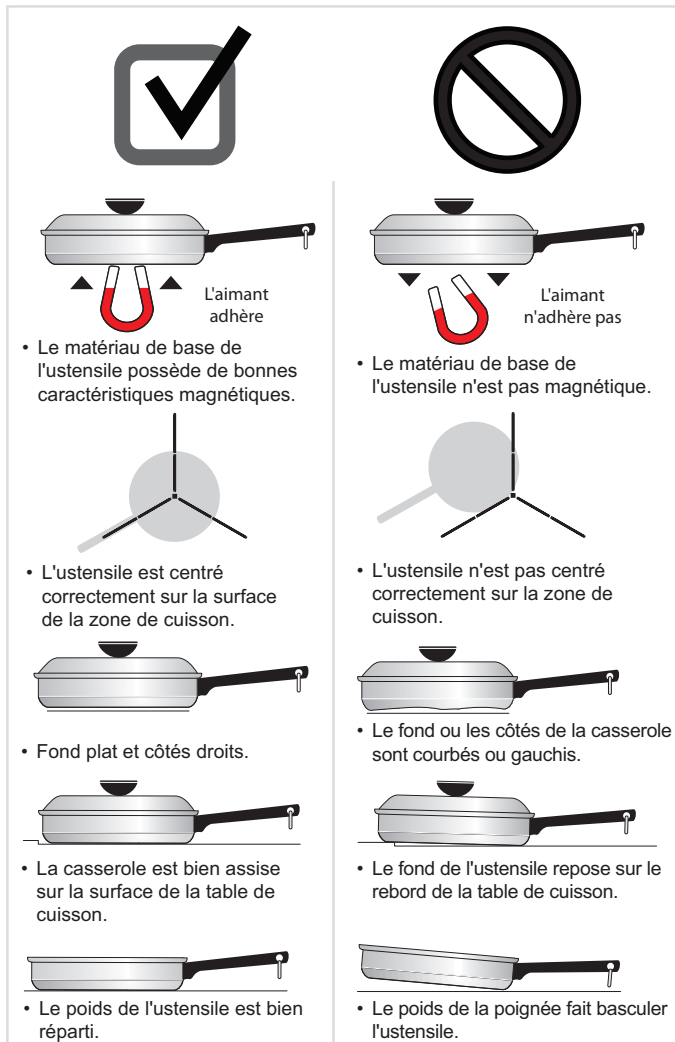
Figure 6 : Détection de l'état de l'ustensile
