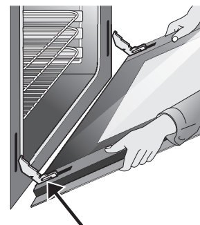
Figure 43 : Maintien de la porte pour le retrait
