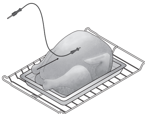
Figure 28 : Positionnement correct de la sonde
