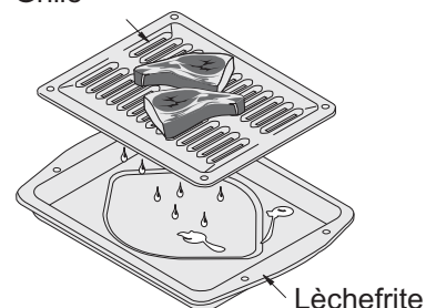
Figure 24 : Lèchefrite et grille
