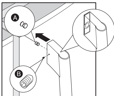
Installation d'un appareil non jumelé
