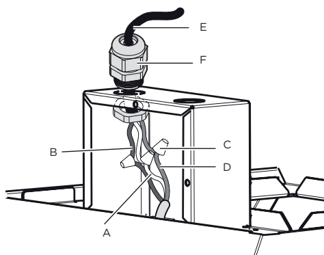
A. Cables blancos B. Cables negros C. Conector de cables (aprobado por UL) D. Cable verde, desnudo o verde/amarillos E. Cable de alimentación eléctrica F. Sujeta cable de 1/2" (aprobado por UL o CSA)
