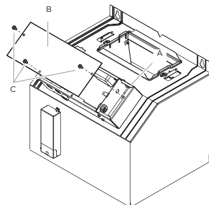
A. Precorte removible B. Cubierta de la caja eléctrica C. Caja eléctrica
