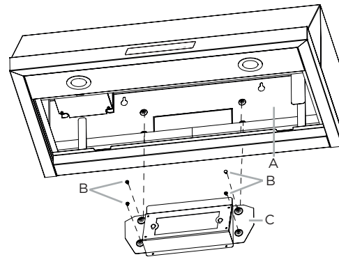
A. Campana (vista interna) B. Tornillos de 4 x 8 mm (4) C. Estufa de montaje del motor
