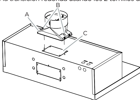
A. Transición redonda superior B. Tornillos de montaje para transición redonda superior (2) C. Cubierta superior removable
