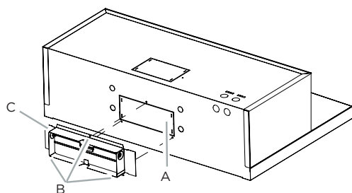
A. Cubierta posterior removable B. Tornillos de montaje para transición rectangular superior (3) C. Transición rectangular posterior
