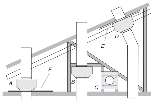
A. Montage au-dessus des solive B. Montage sur traverses de ferme
