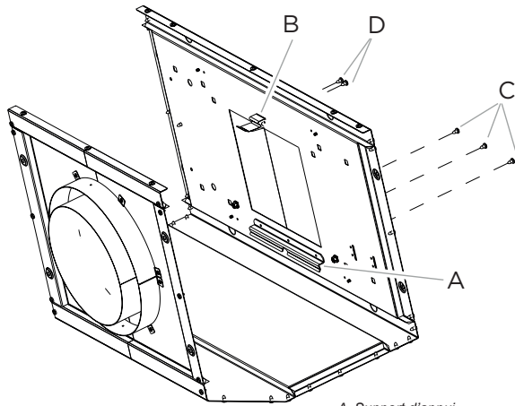
A. Support d'appui B. Languette de ressort C. 3 vis de 4,2 x 8 mm D. 2 vis de 4,2 x 8 mm
