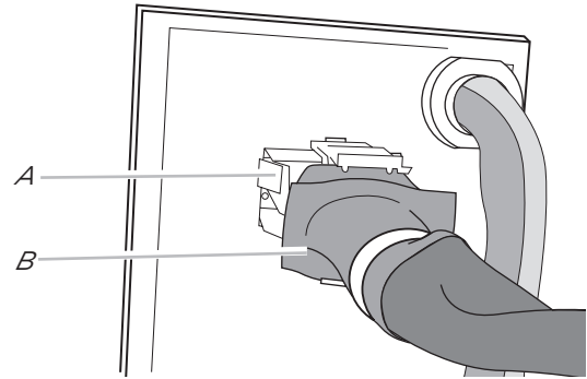
A. Conector de la caja de conexiones B. cable de alimentación de la campana
