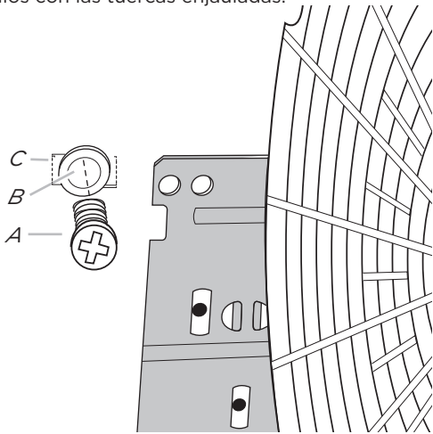
A. Tornillo de 6 x 16 mm B. Arandela C. Tuerca enjaulada
