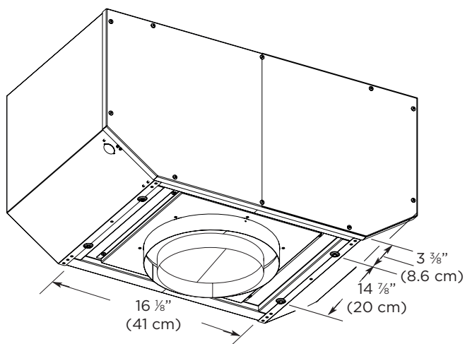
VUE DE DESSOUS (ENTRÉE)
