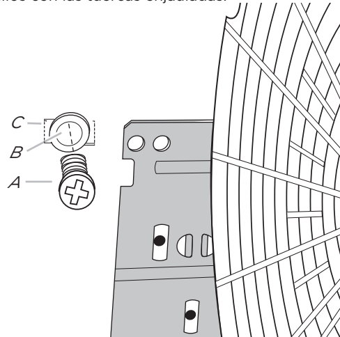
A. Tornillo de 6 x 16 mm B. Arandela C. Tuercas enjauladas
