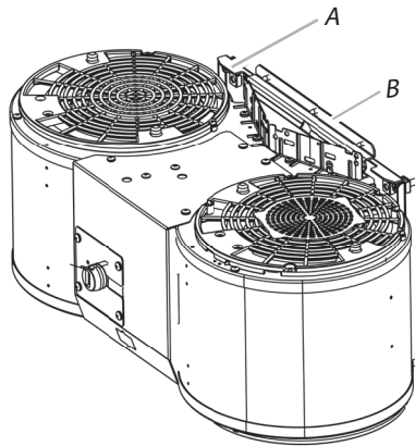
A. Plato de montaje del motor B. Soporte de montaje del motor
