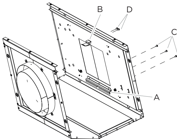
A. Soporte de montaje B. Clip de soporte C. Tornillos 3 - 4.2 x 8 mm D. Tornillos 2 - 4.2 x 8 m
