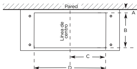
DIMENSIONES DEL HOUSING SUPERIOR DE MOTOR
