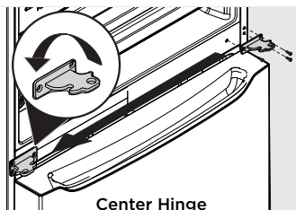
Center Hinge
