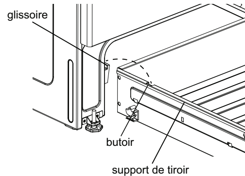
Figure 23 : Composants du tiroir de rangement
