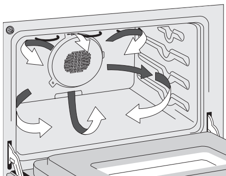
Circulation d'air chaud lors de la cuisson par convection Figure 1
