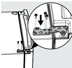
Charnière supérieure
