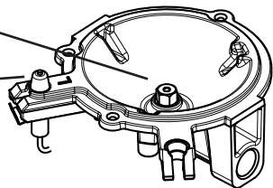
Figure 1: Chapeau de brûleur, tête de brûleur, allumeur et orifice
