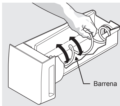
Ajuste de la barrena del compartimento para hielo
