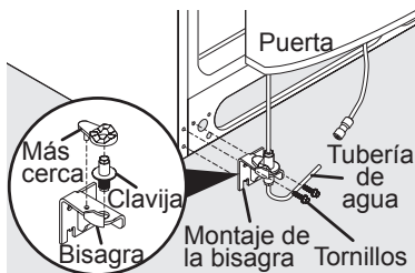
Bisagra ajustable (algunos modelos)
