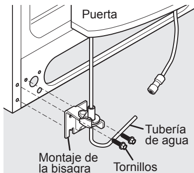
Bisagra no ajustable (algunos modelos)
