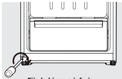
Fije la bisagra inferior
