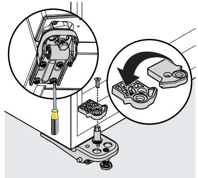
Door Stopper
