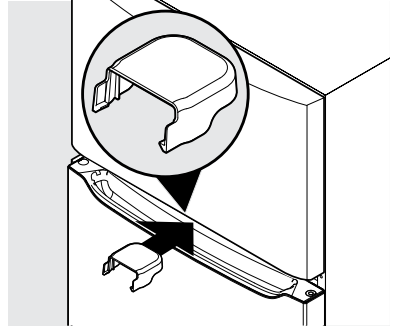
Level Door
