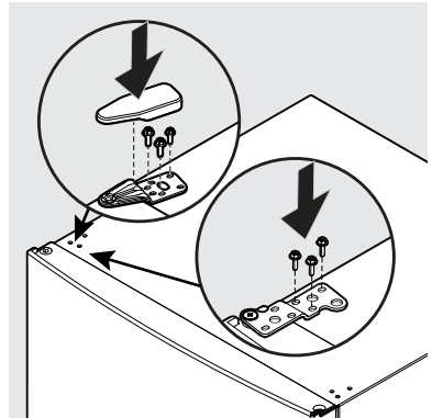
Top Hinge
