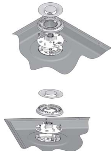
VISTA DE DESPIEZO DEL QUEMADOR
