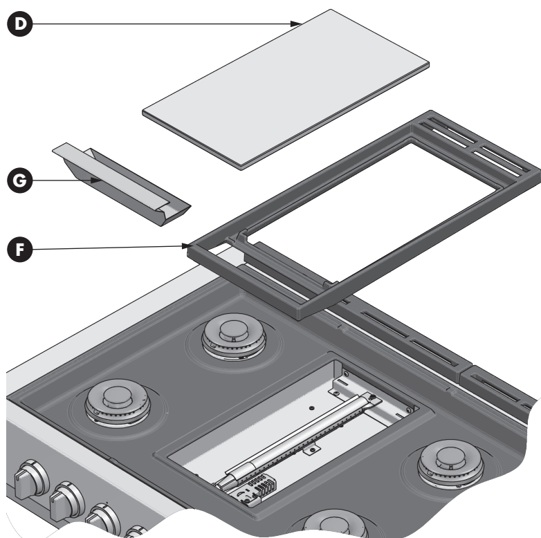
D - Plaque de gril G - Bac d'égouttement F - Support de plaque de gril
