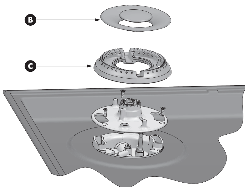
B - Brûleur coupe C - Épandeur Gas Burners
